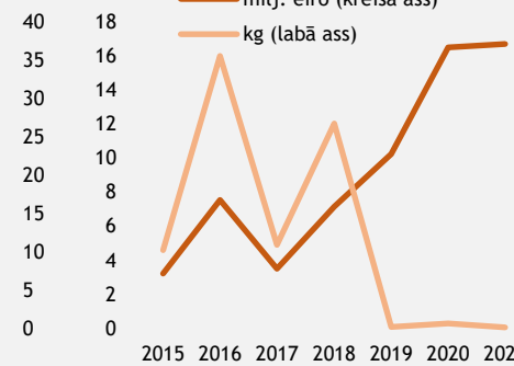
Heterocikliskie savienojumi
