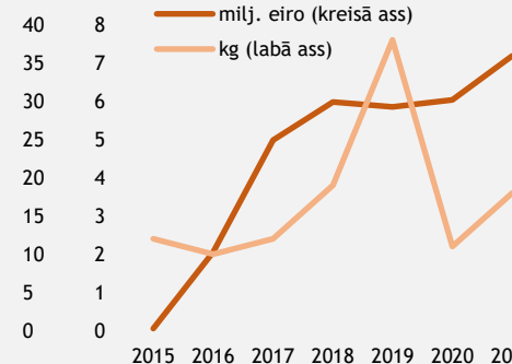
Heterocikliskie savienojumi
