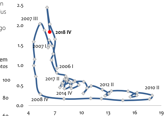
Beveridža likne Latvijā Procentos pa ceturkšņiem, vertikālā ass – vakanču skaits pret ekonomiski aktīviem iedzīvotājiem; horizontālā ass – bezdarba līmenis
